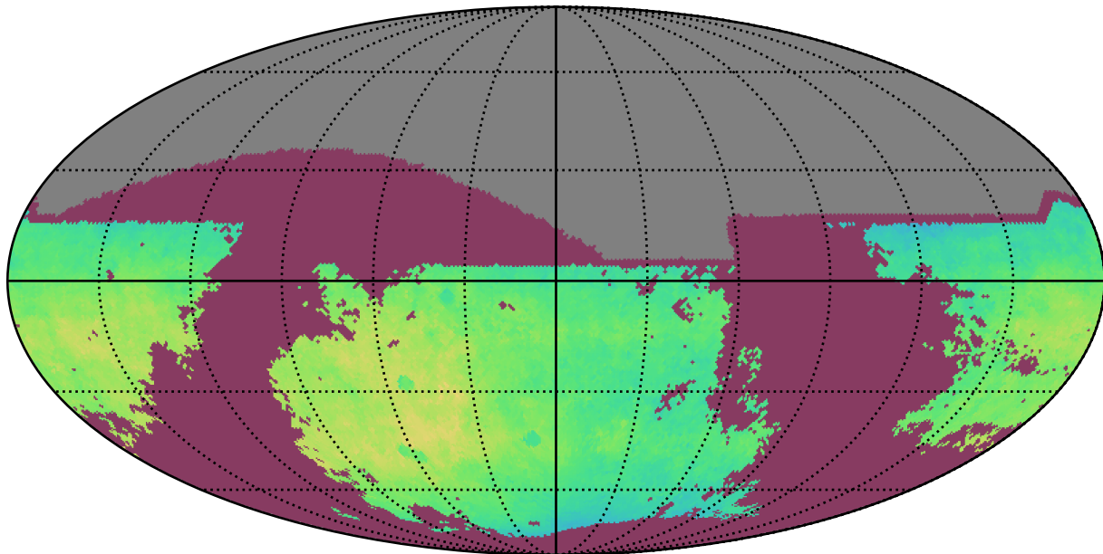
reweight_bulge_v3.3_10yrs i: NgalScale
