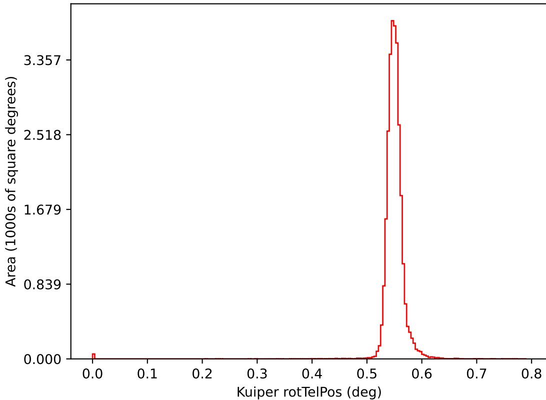
reweight_bulge_v3.3_10yrs i: Kuiper rotTelPos
