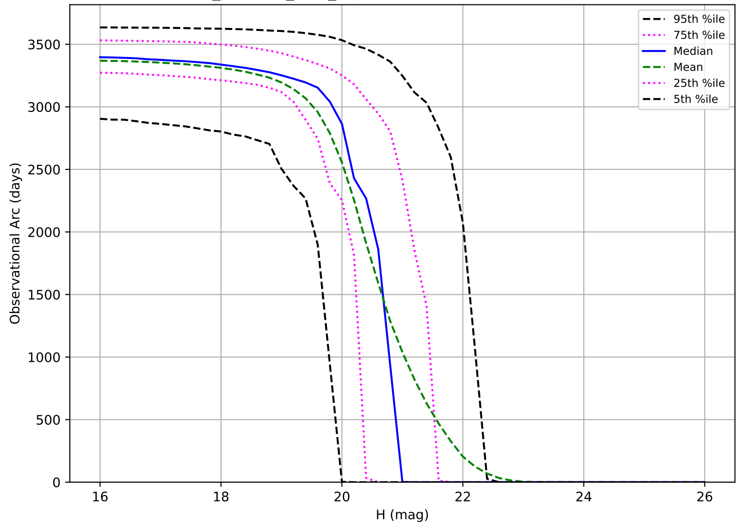
retro_baseline_v2.0_10yrs: Observational Arc Length MBA
