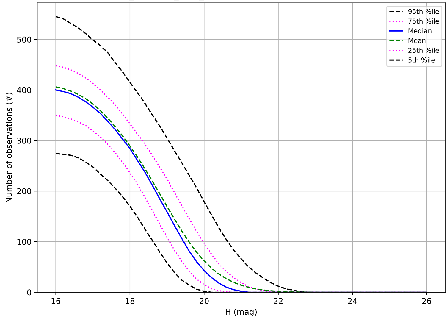
retro_baseline_v2.0_10yrs: Number of observations MBA
