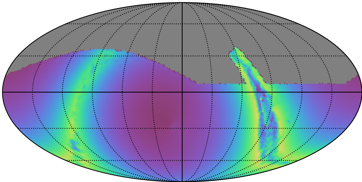
retro_baseline_v2.0_10yrs : young_stars
