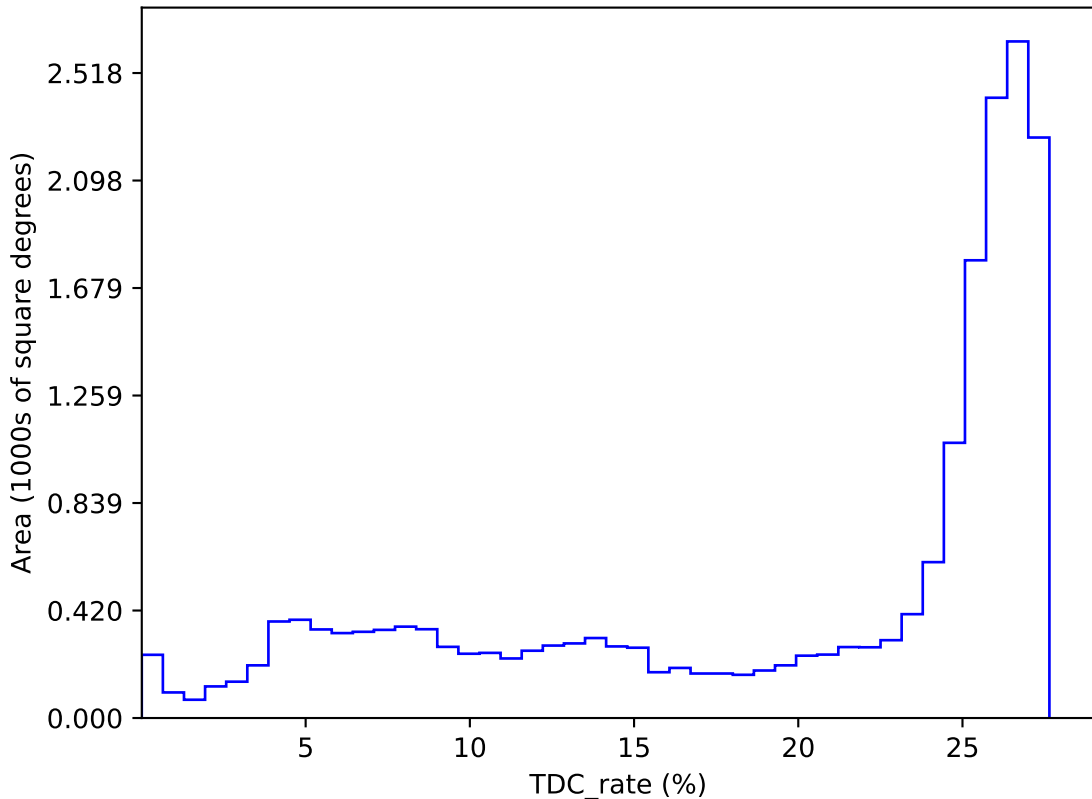
retro_baseline_v2.0_10yrs : TDC_rate
