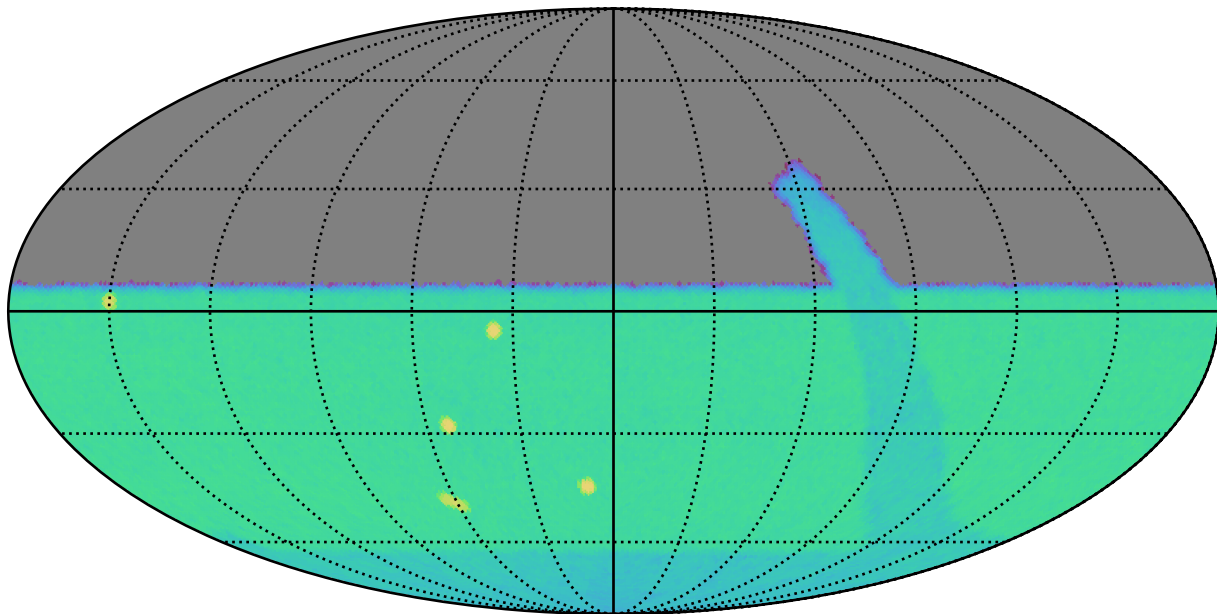
retro_baseline_v2.0_10yrs u: SurfaceBrightLimit
