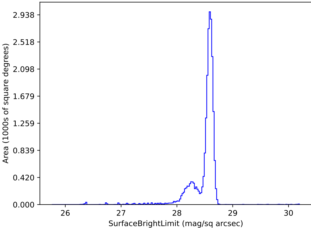
retro_baseline_v2.0_10yrs u: SurfaceBrightLimit
