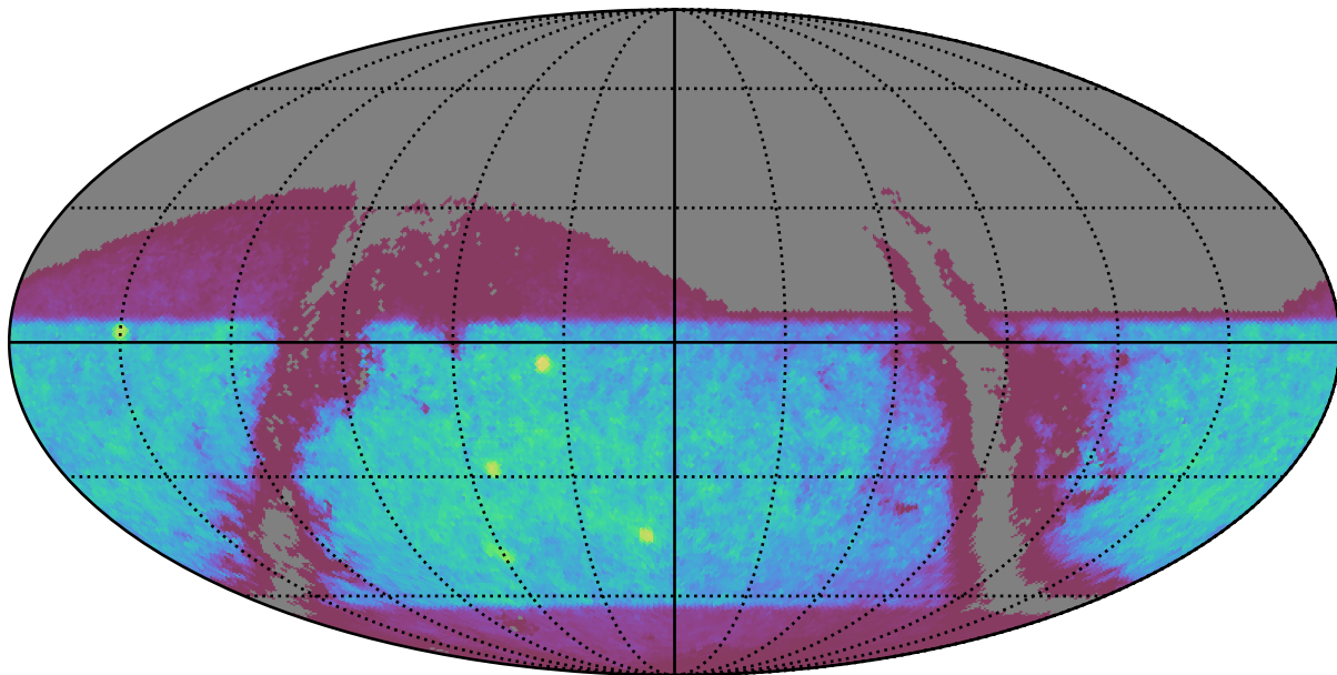
retro_baseline_v2.0_10yrs : SNSLMetric
