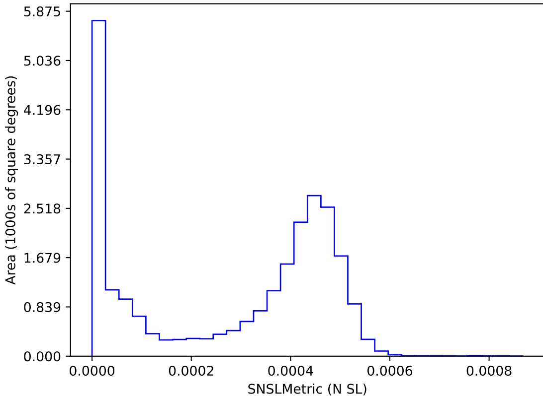
retro_baseline_v2.0_10yrs : SNSLMetric
