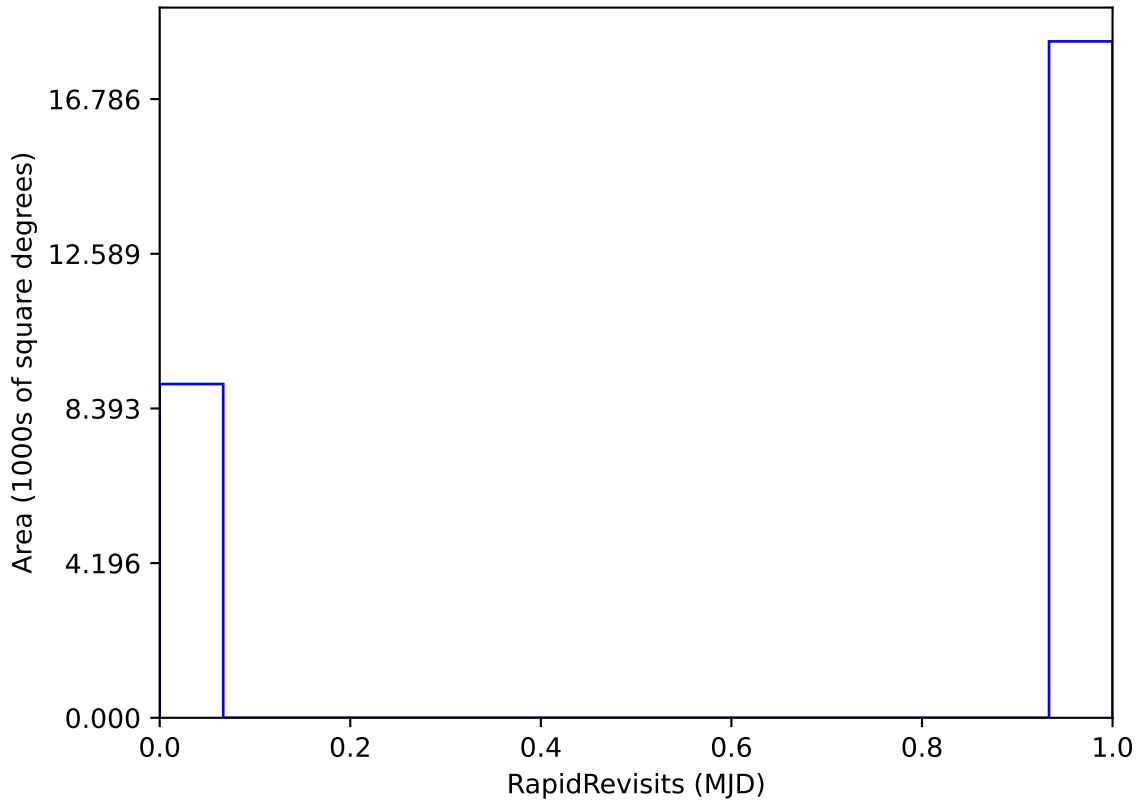
retro_baseline_v2.0_10yrs : RapidRevisits
