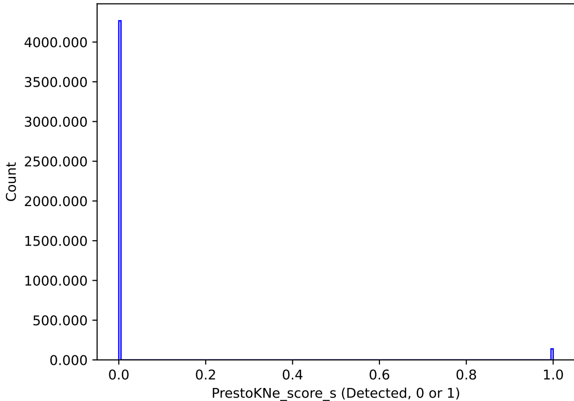
retro_baseline_v2.0_10yrs : PrestoKNe_score_s
