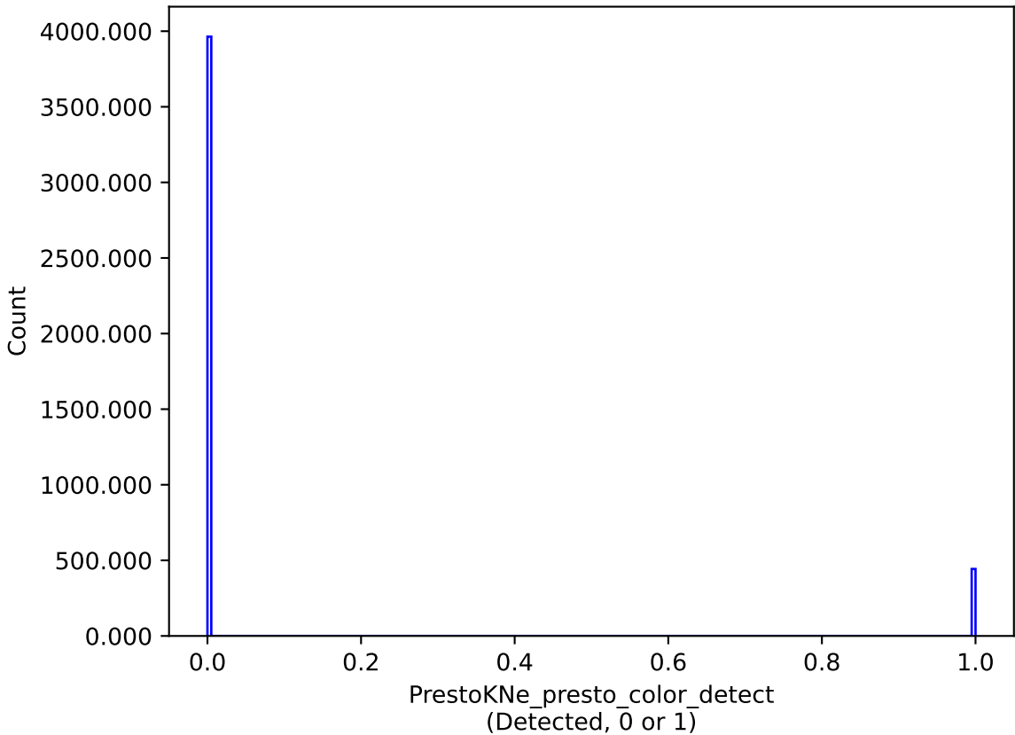
retro_baseline_v2.0_10yrs : PrestoKNe_presto_color_detect
