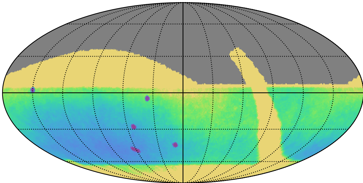
retro_baseline_v2.0_10yrs : Parallax Uncert @ 24.0
