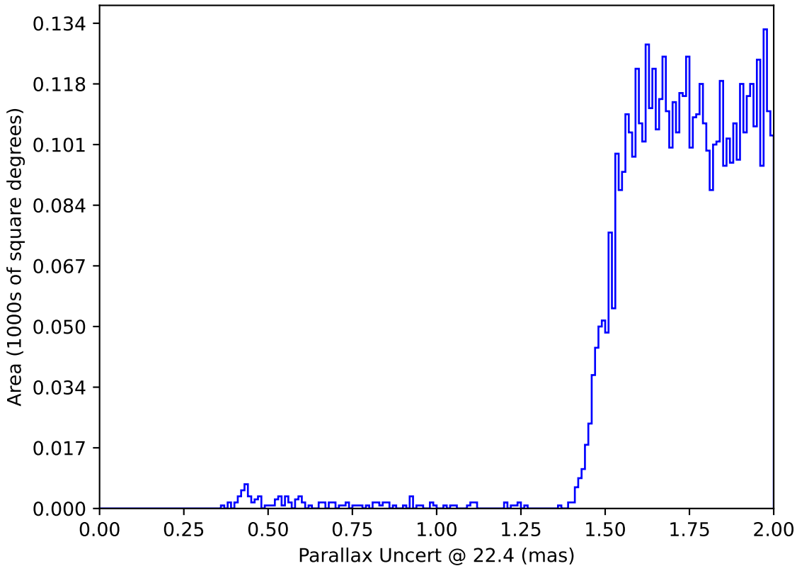
retro_baseline_v2.0_10yrs : Parallax Uncert @ 22.4
