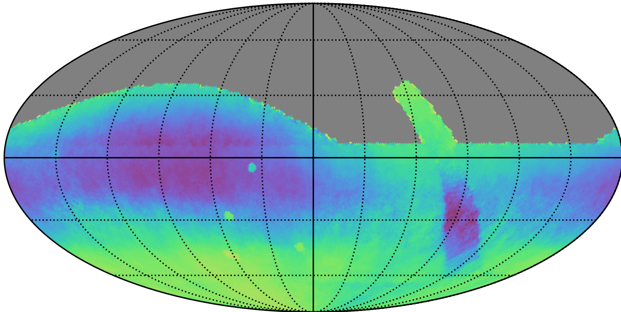
retro_baseline_v2.0_10yrs : Parallax-DCR degeneracy @ 24.0
