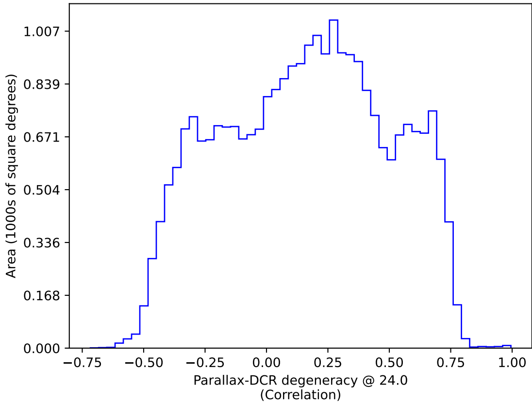
retro_baseline_v2.0_10yrs : Parallax-DCR degeneracy @ 24.0
