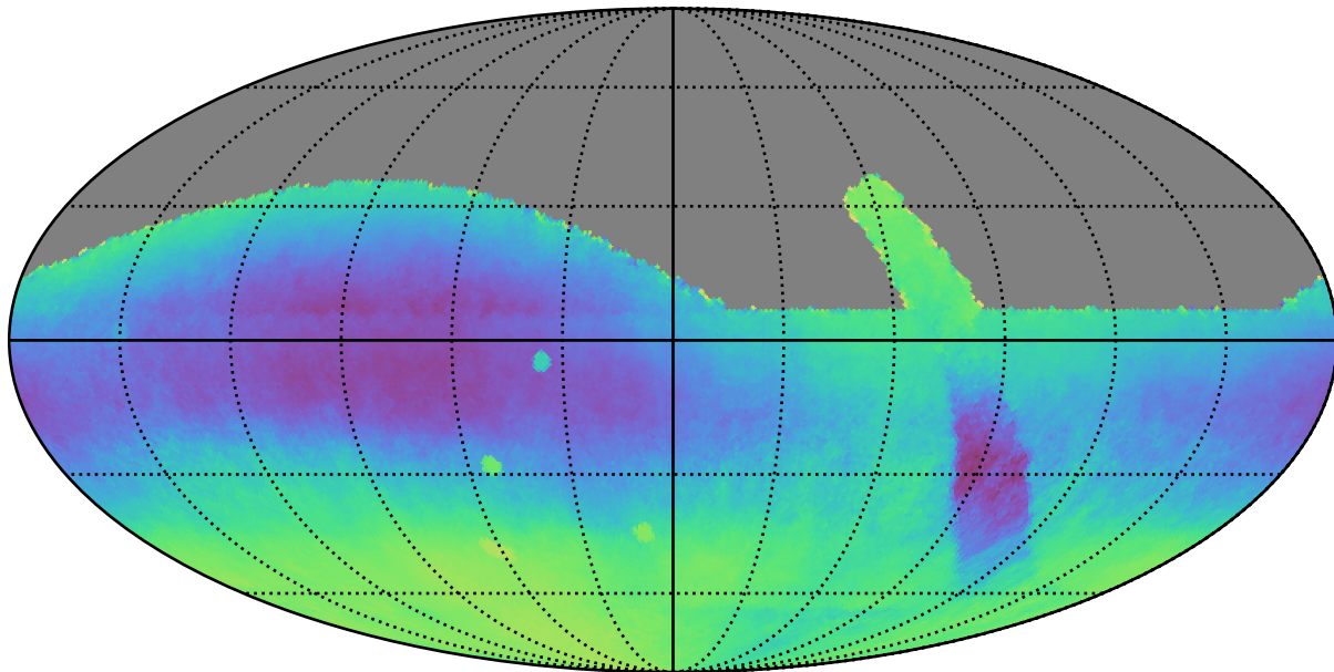
retro_baseline_v2.0_10yrs : Parallax-DCR degeneracy @ 22.4
