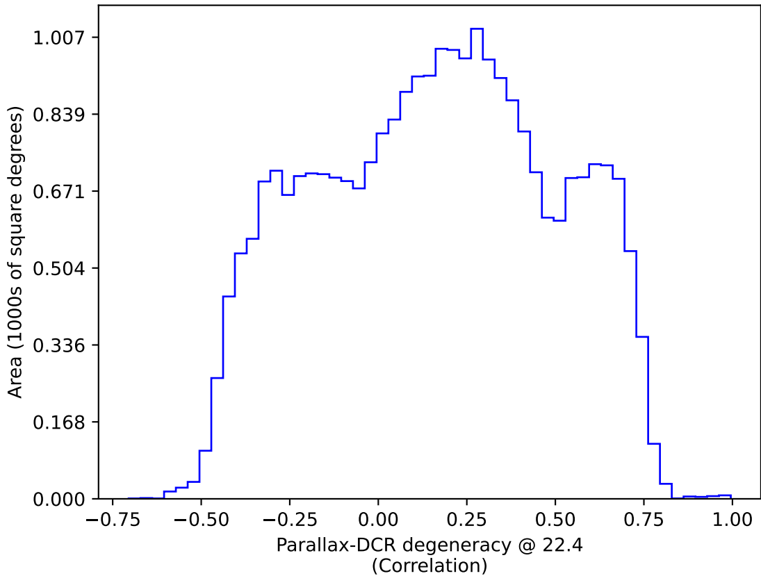
retro_baseline_v2.0_10yrs : Parallax-DCR degeneracy @ 22.4
