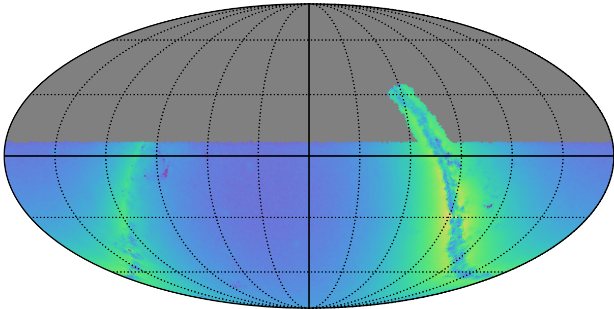
retro_baseline_v2.0_10yrs u: Nstars_no_crowding
