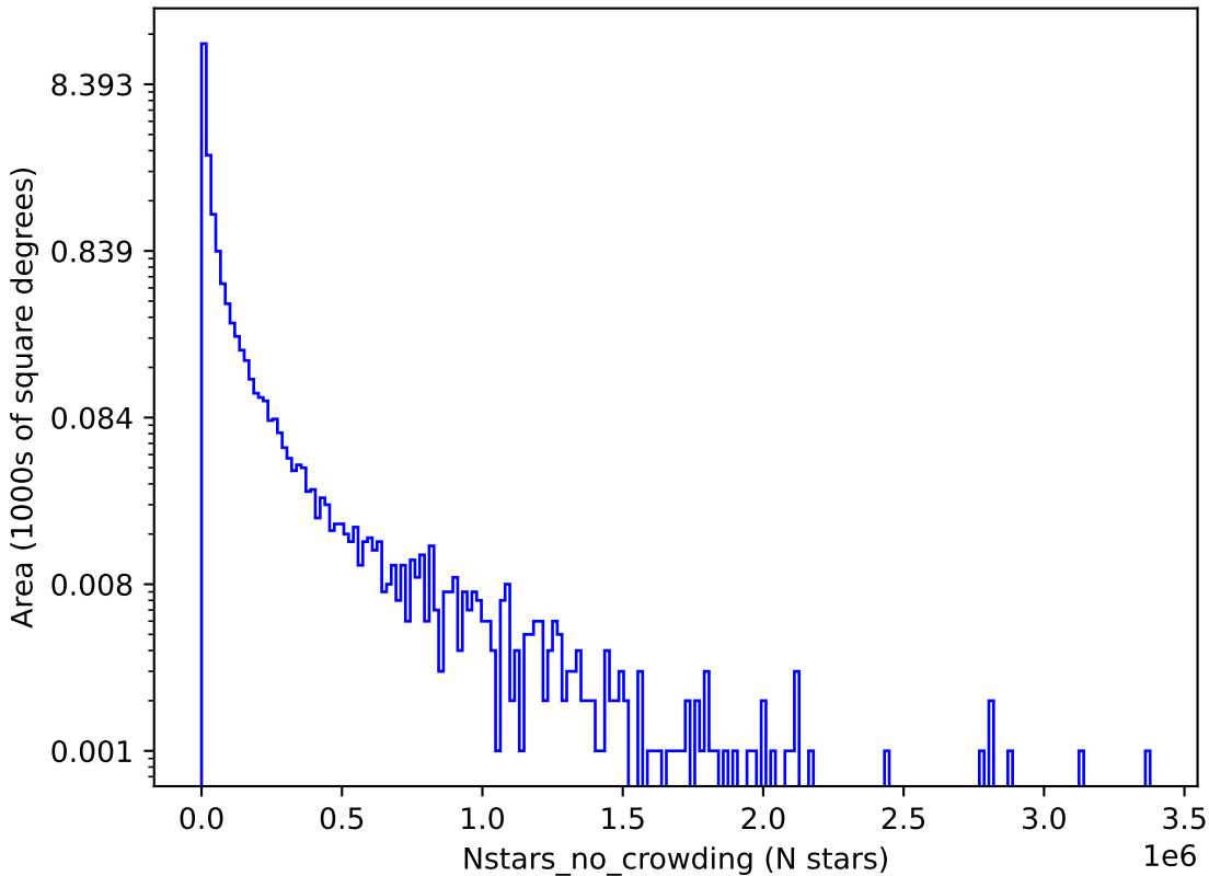
retro_baseline_v2.0_10yrs u: Nstars_no_crowding
