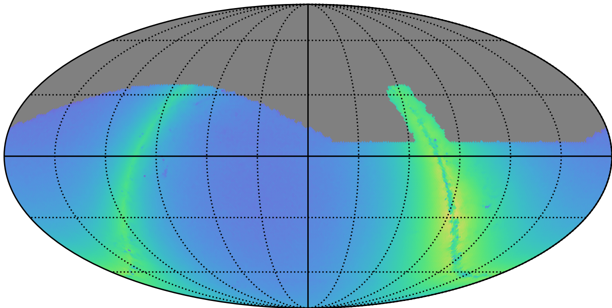
retro_baseline_v2.0_10yrs i: Nstars_no_crowding
