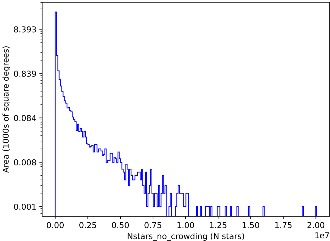
retro_baseline_v2.0_10yrs i: Nstars_no_crowding
