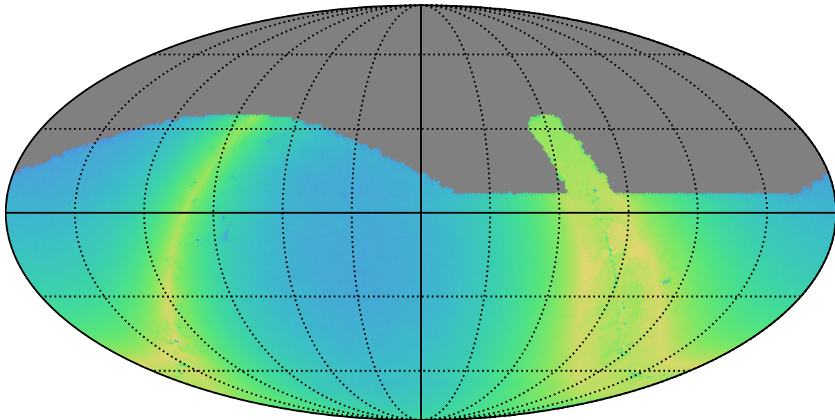
retro_baseline_v2.0_10yrs z: N stars to Precision 0.20
