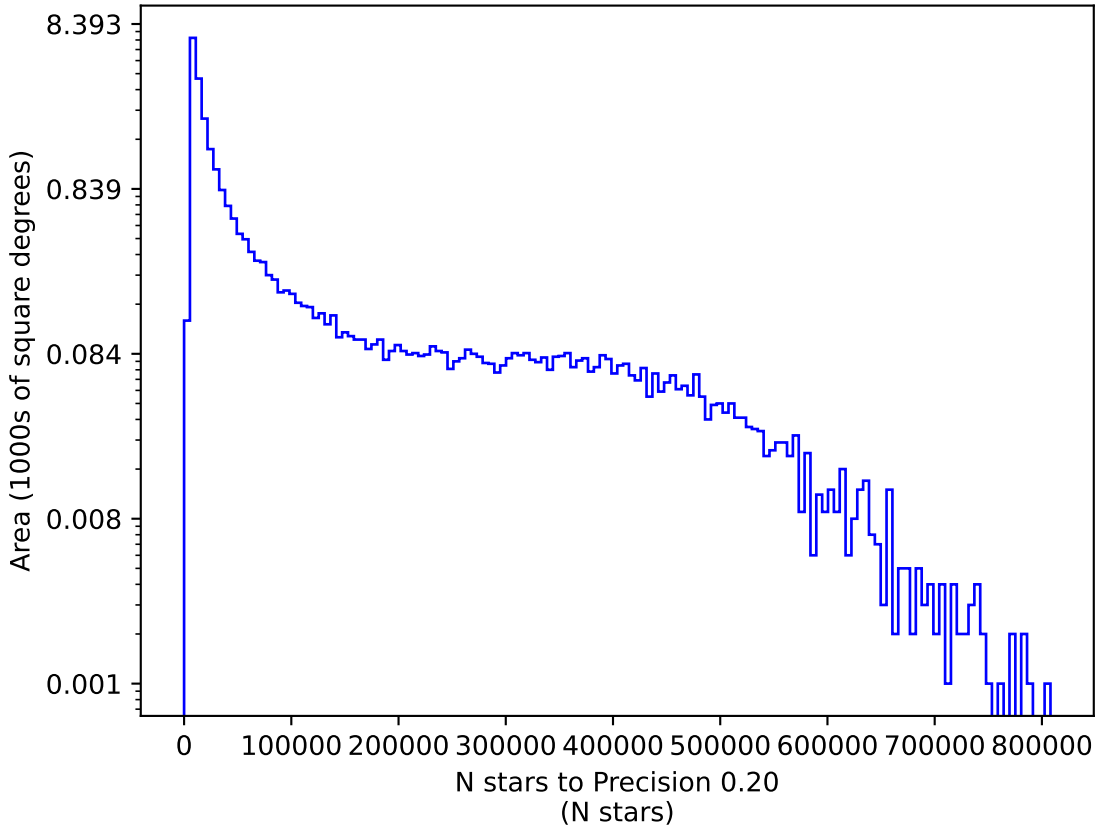
retro_baseline_v2.0_10yrs z: N stars to Precision 0.20
