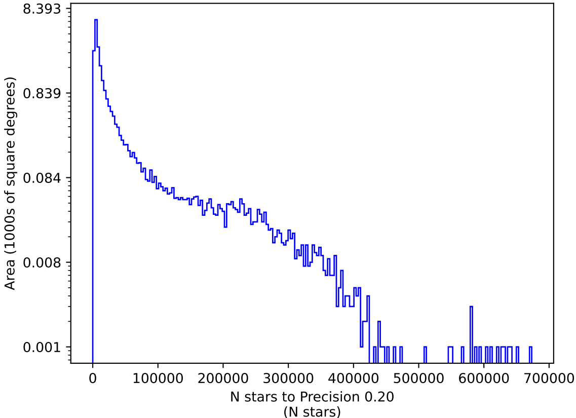
retro_baseline_v2.0_10yrs u: N stars to Precision 0.20
