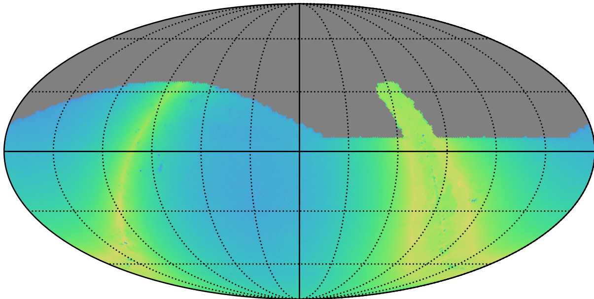
retro_baseline_v2.0_10yrs i: N stars to Precision 0.20
