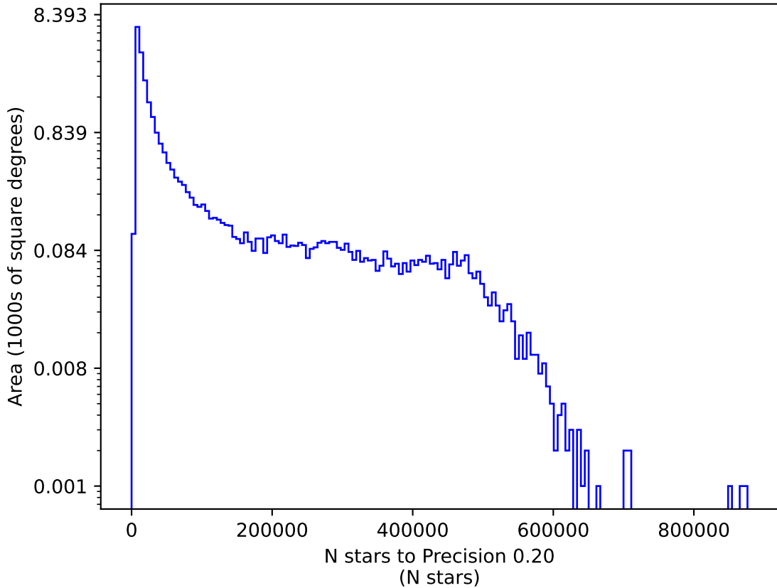
retro_baseline_v2.0_10yrs i: N stars to Precision 0.20
