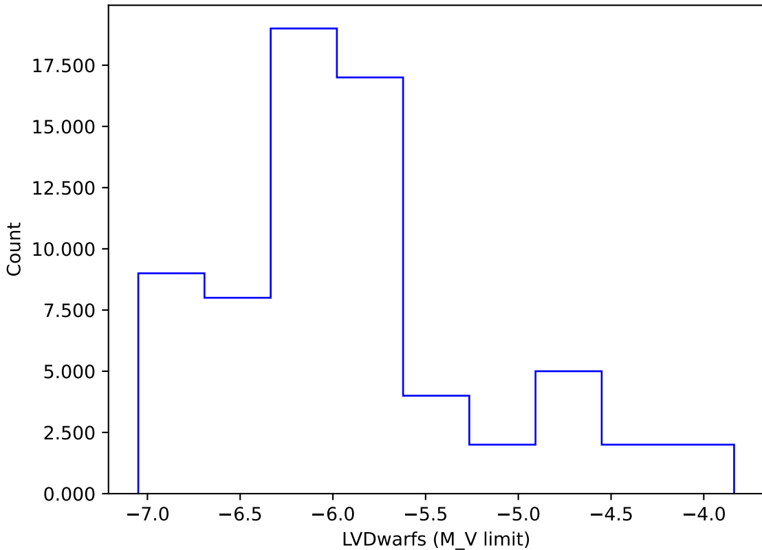
retro_baseline_v2.0_10yrs gi: LVDwarfs
