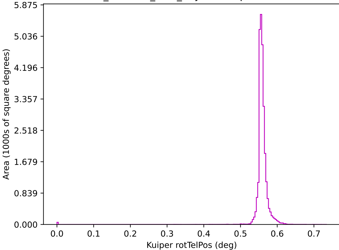
retro_baseline_v2.0_10yrs z: Kuiper rotTelPos
