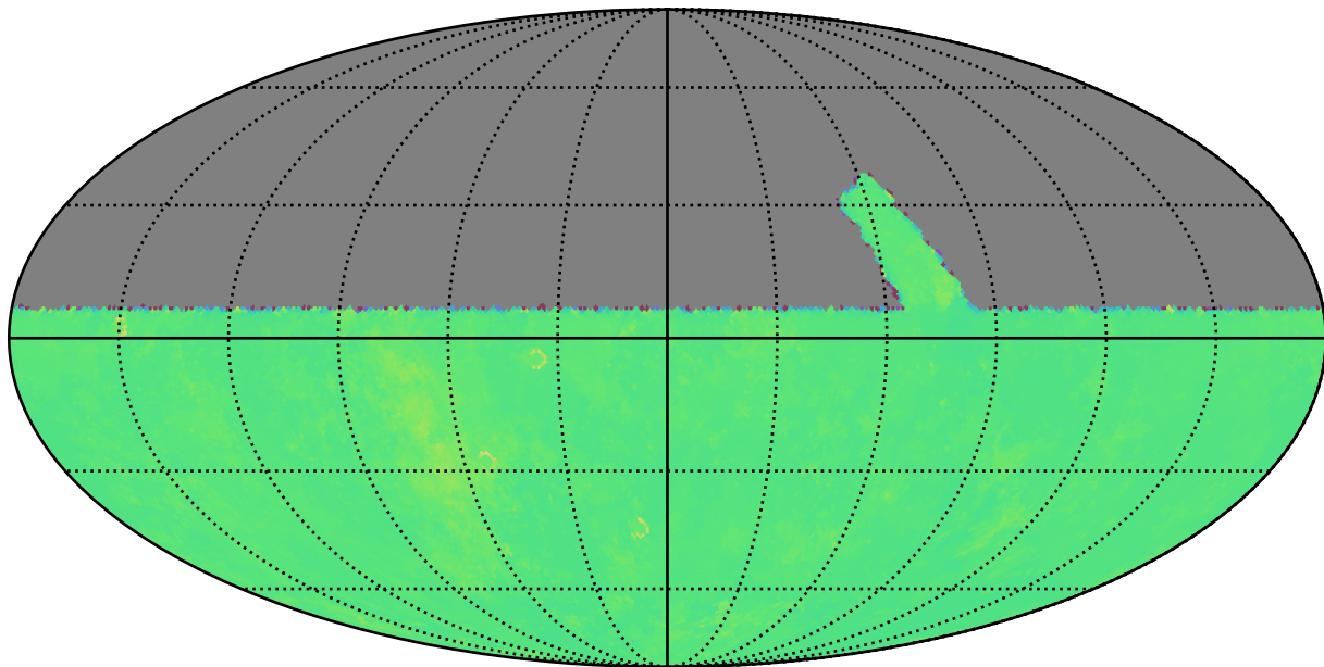
retro_baseline_v2.0_10yrs u: Kuiper rotTelPos
