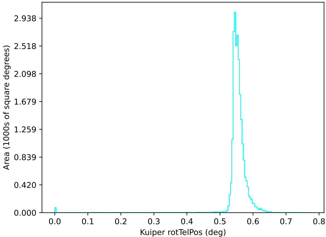
retro_baseline_v2.0_10yrs u: Kuiper rotTelPos
