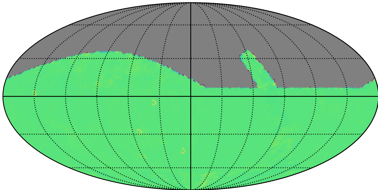
retro_baseline_v2.0_10yrs r: Kuiper rotTelPos
