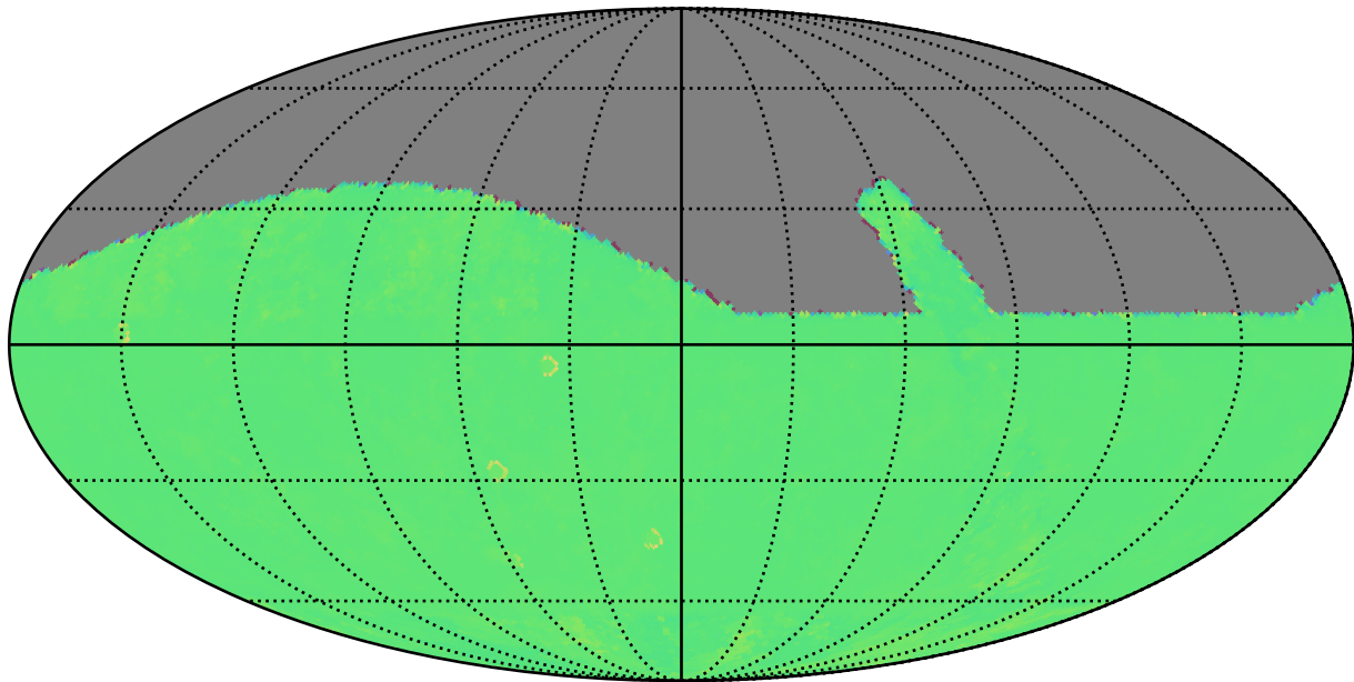
retro_baseline_v2.0_10yrs i: Kuiper rotTelPos
