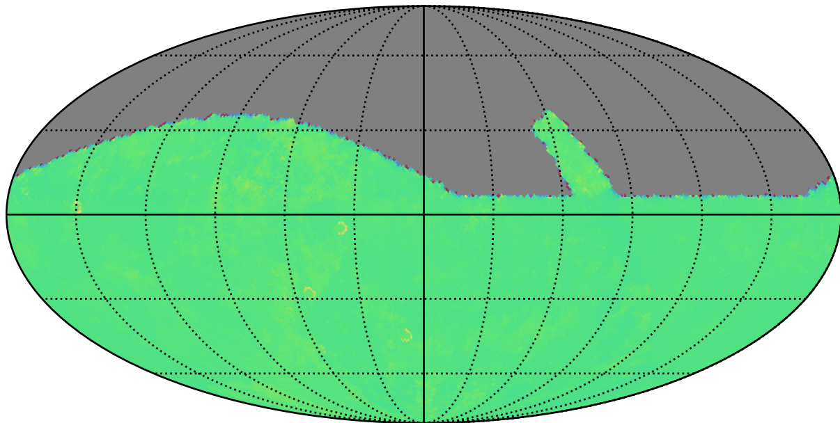
retro_baseline_v2.0_10yrs g: Kuiper rotTelPos
