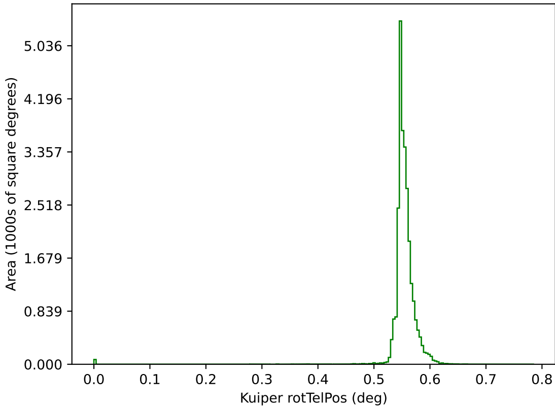
retro_baseline_v2.0_10yrs g: Kuiper rotTelPos
