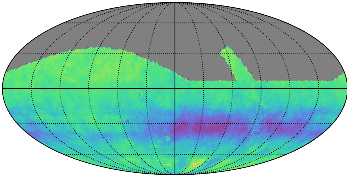
retro_baseline_v2.0_10yrs z: Kuiper rotSkyPos
