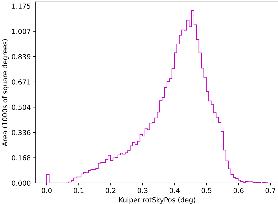
retro_baseline_v2.0_10yrs z: Kuiper rotSkyPos
