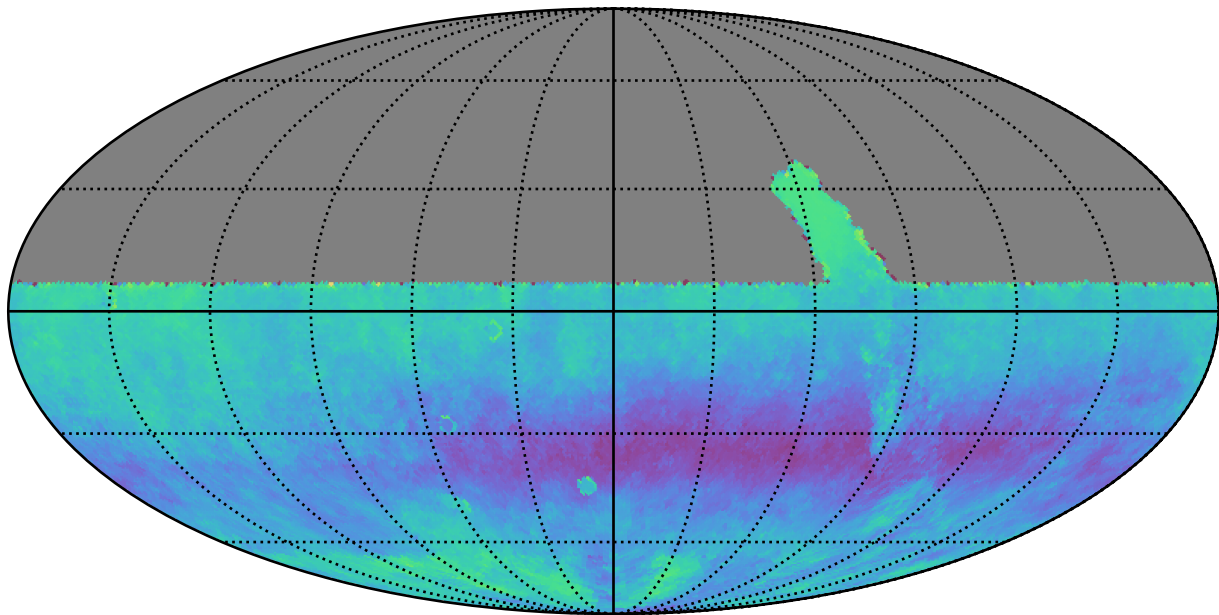
retro_baseline_v2.0_10yrs y: Kuiper rotSkyPos
