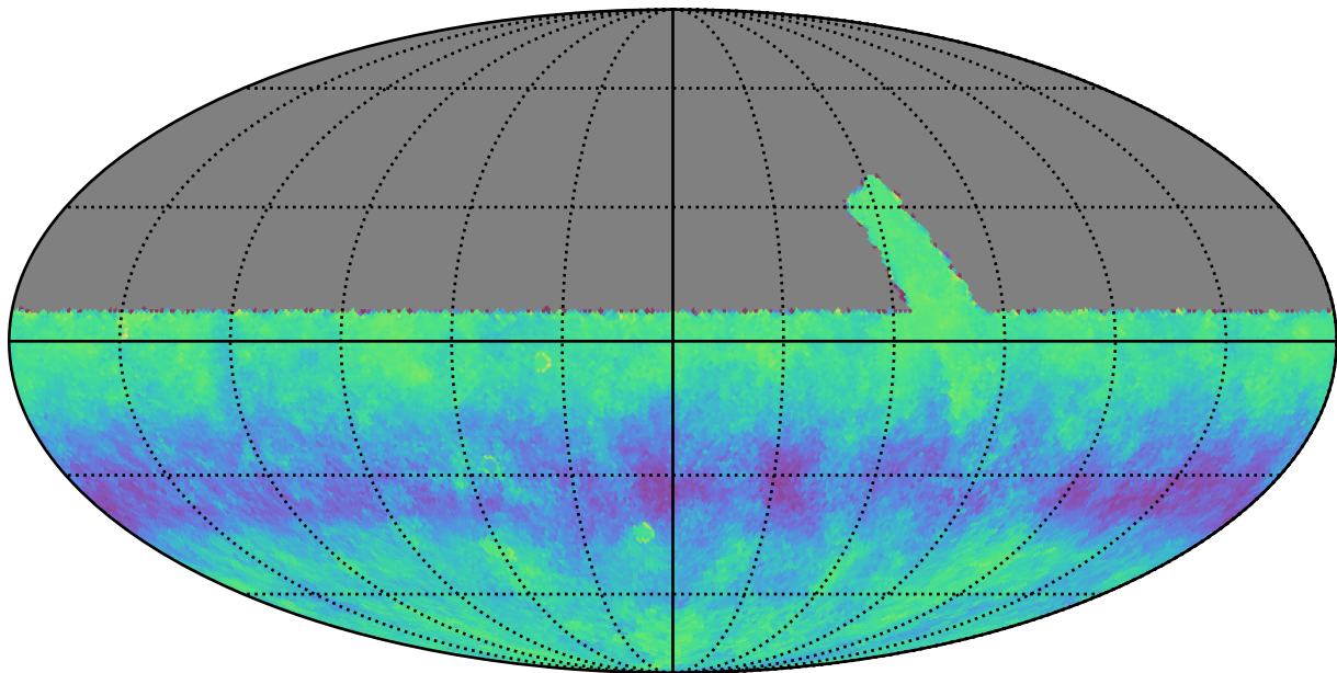
retro_baseline_v2.0_10yrs u: Kuiper rotSkyPos
