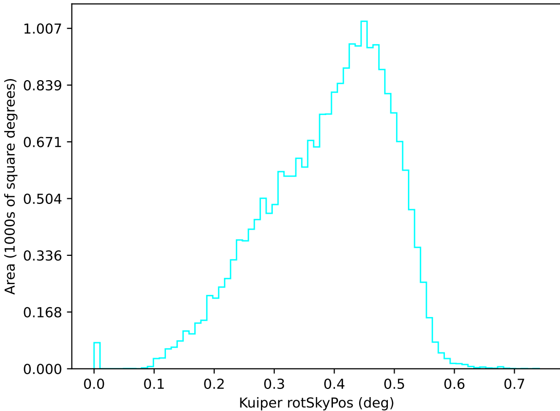
retro_baseline_v2.0_10yrs u: Kuiper rotSkyPos
