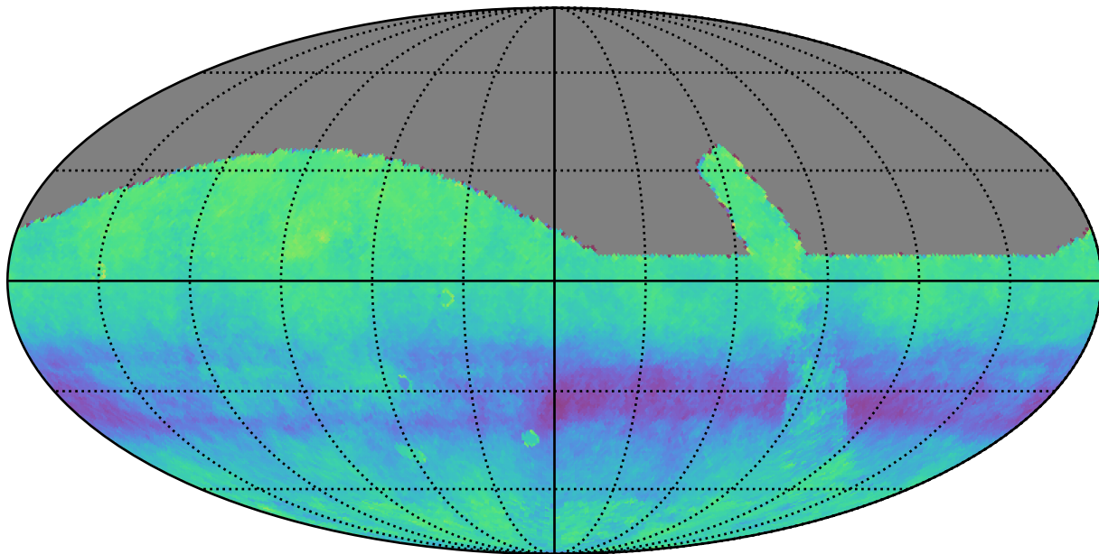
retro_baseline_v2.0_10yrs r: Kuiper rotSkyPos
