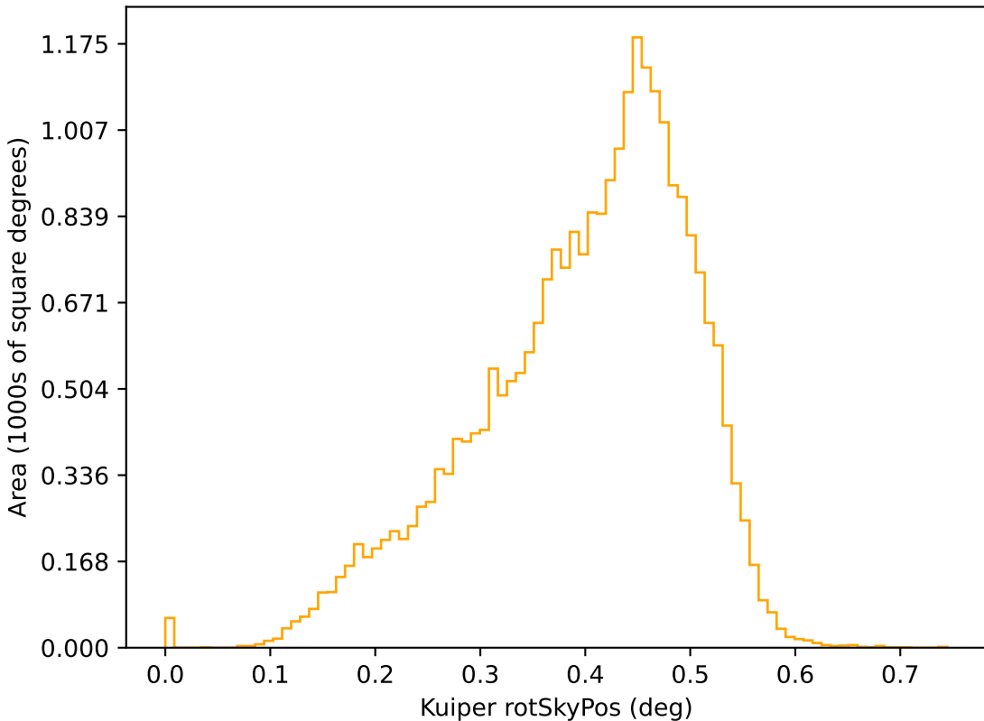
retro_baseline_v2.0_10yrs r: Kuiper rotSkyPos
