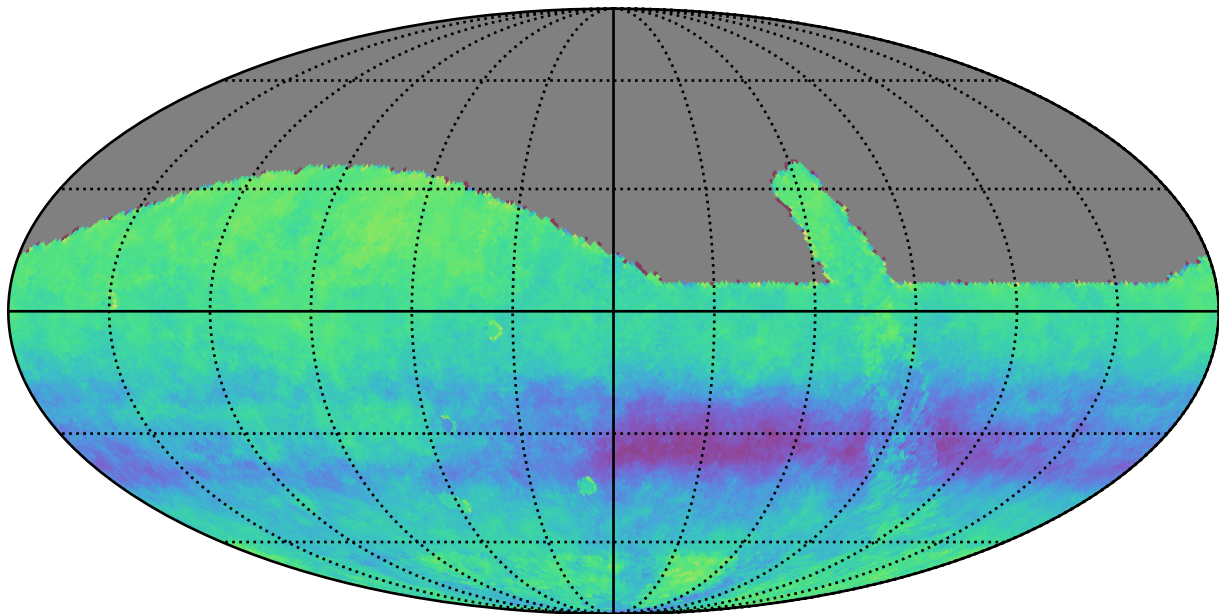
retro_baseline_v2.0_10yrs i: Kuiper rotSkyPos
