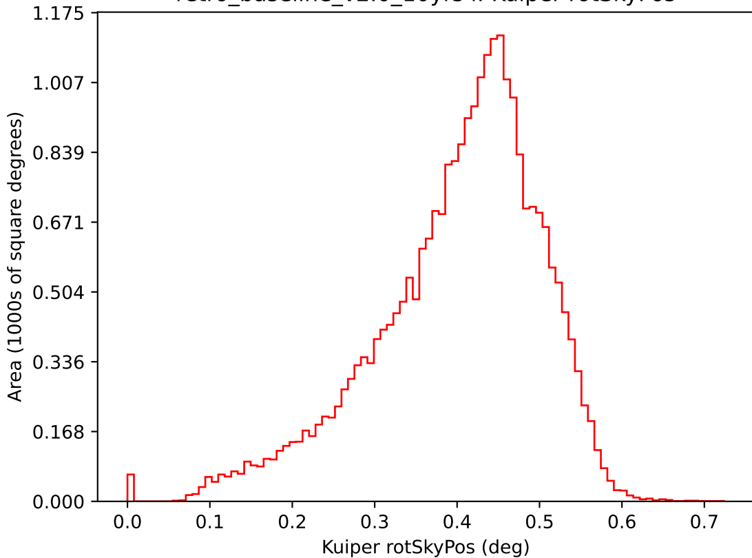
retro_baseline_v2.0_10yrs i: Kuiper rotSkyPos
