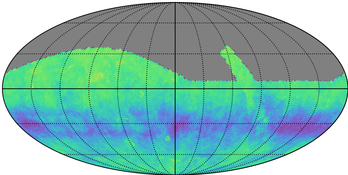
retro_baseline_v2.0_10yrs g: Kuiper rotSkyPos
