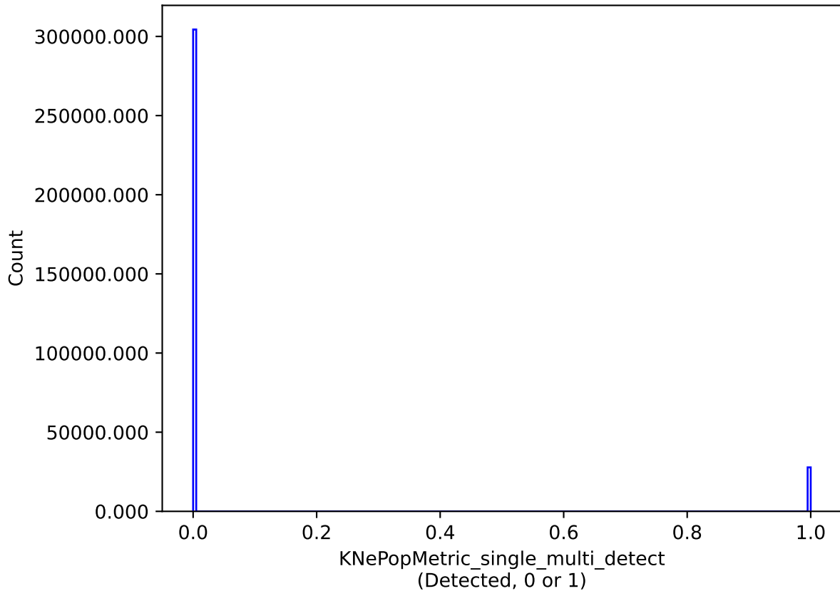
retro_baseline_v2.0_10yrs single model: KNePopMetric_single_multi_detect
