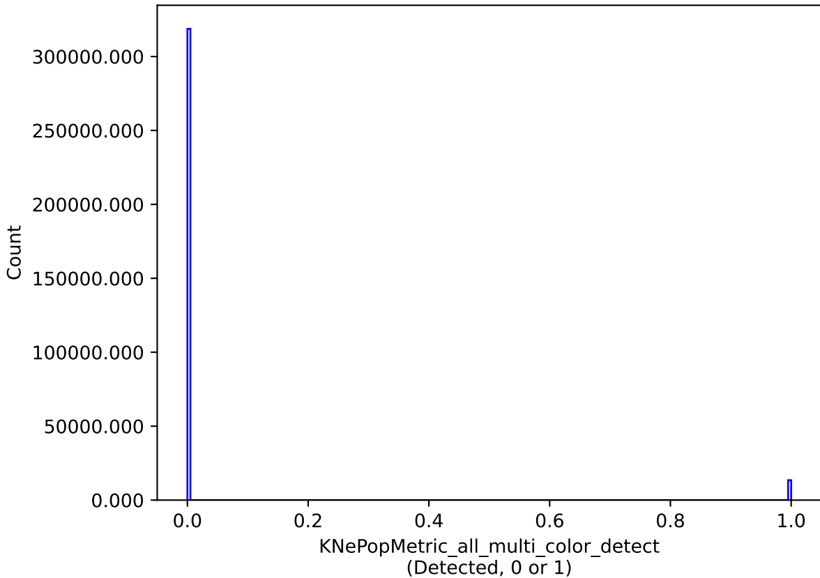
retro_baseline_v2.0_10yrs all models: KNePopMetric_all_multi_color_detect
