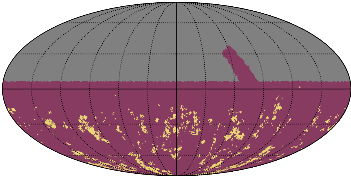
retro_baseline_v2.0_10yrs u band: Gaps_7hr
