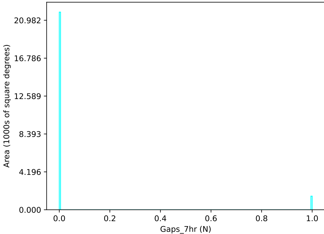
retro_baseline_v2.0_10yrs u band: Gaps_7hr
